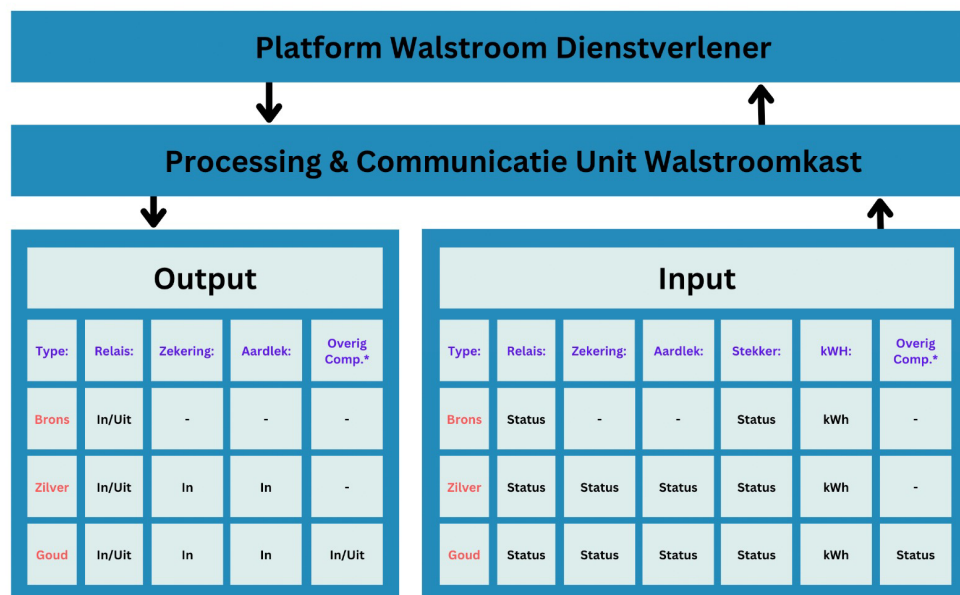
Afbeelding 1: schematische weergave functionaliteiten type walstroomkasten.
